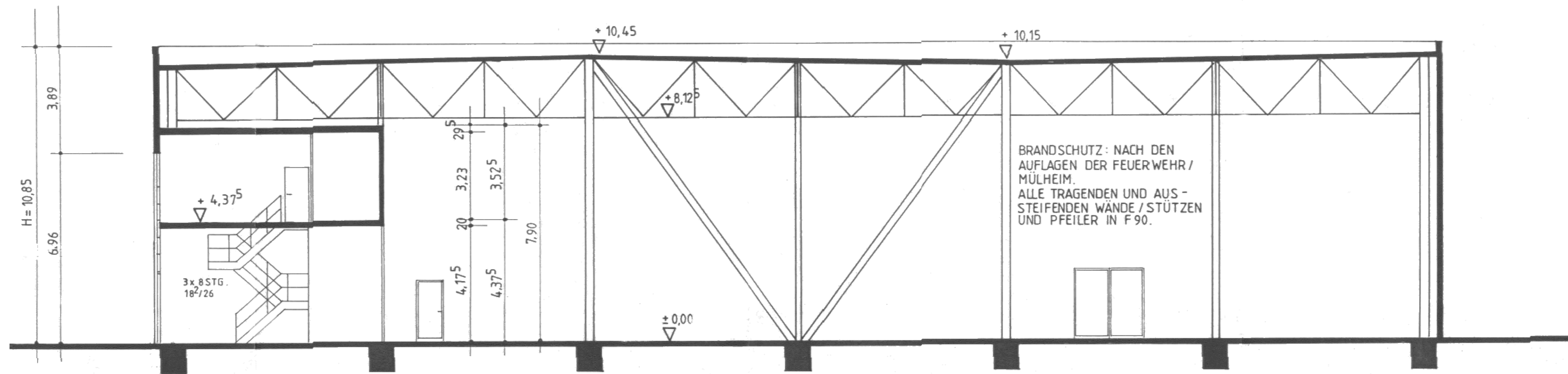
QUERSCHNITT A-A BESTEHENDES GEBÄUDE
